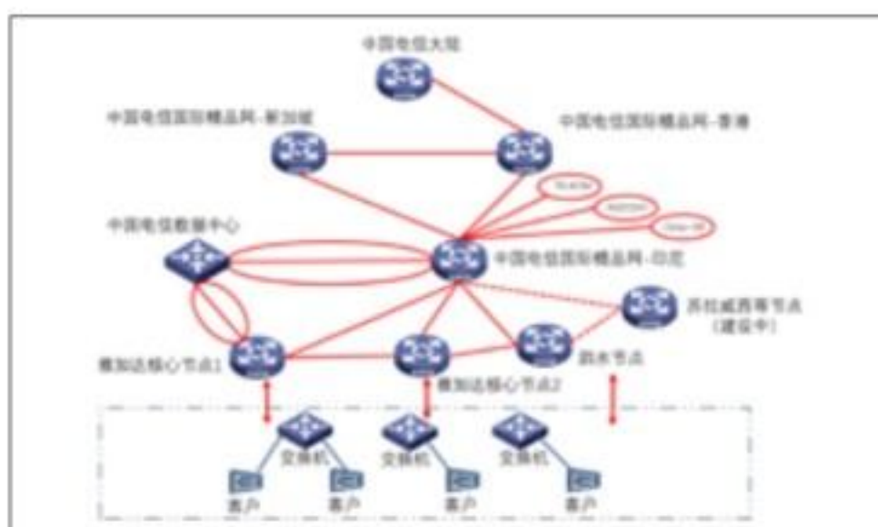
中国电信印尼 IP 网络架构图 提供回国精品互联网
